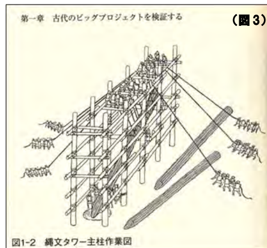
図1-2 縄文タワー主柱作業図
